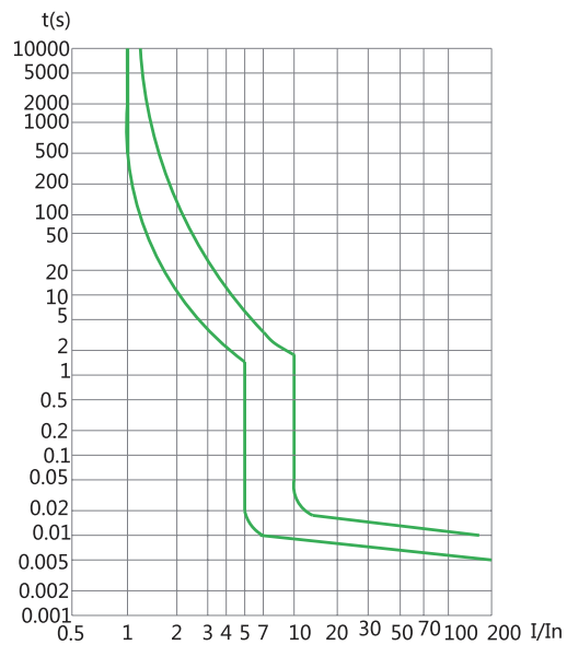
Charakteristika C
