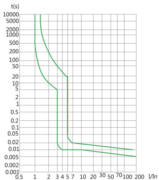
Charakteristika B
