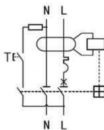
Schéma zapojení
