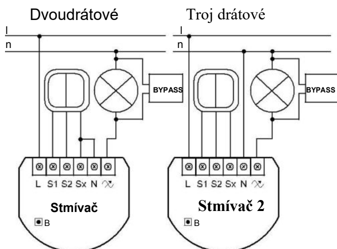
Schéma zapojení 3 zapojení Bypass FGB-002
