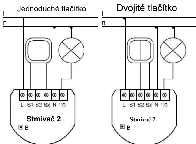
schéma zapojení 2: Troj drátové zapojení
