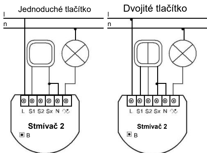
Schéma 1: Dvoudrátové zapojení
