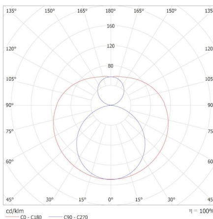
KANLUX S.A. (kat 26065) T8 LED GLASSv3 18W CW / Krzywa rozsyłu światła (biegunowo)
