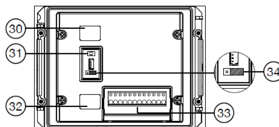
ZADNÍ POHLED
