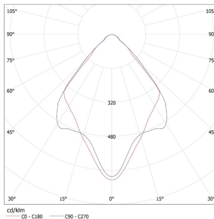
KANLUX S.A. (kat 26738) APRILA DTO-W i PRO GU10 LED 7W / LDC (Polar)
