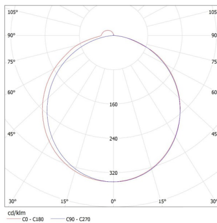
KANLUX S.A. (kat 26682) ASTEN LED IP44-15W-NW / Krzywa rozsyłu światła (biegunowo)
