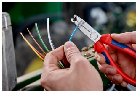
otvory pro odizolování pro vodiče 1,5 mm 2 a 2,5 mm 2
