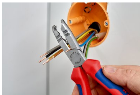
řezání při zkracování jednotlivých vodičů
