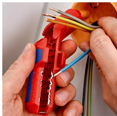
Odizolování jednotlivých vodičů
