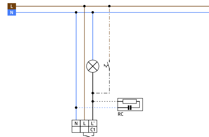
Schéma zapojení
