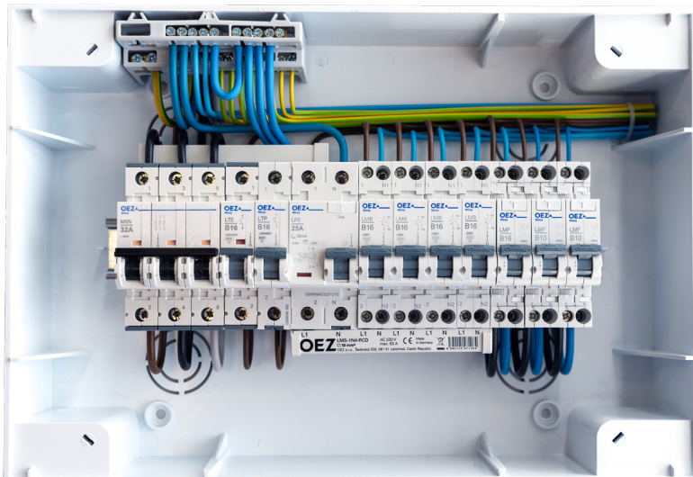
14modulová rozvodnice DBO-RZG-N-1S14-14-090101
