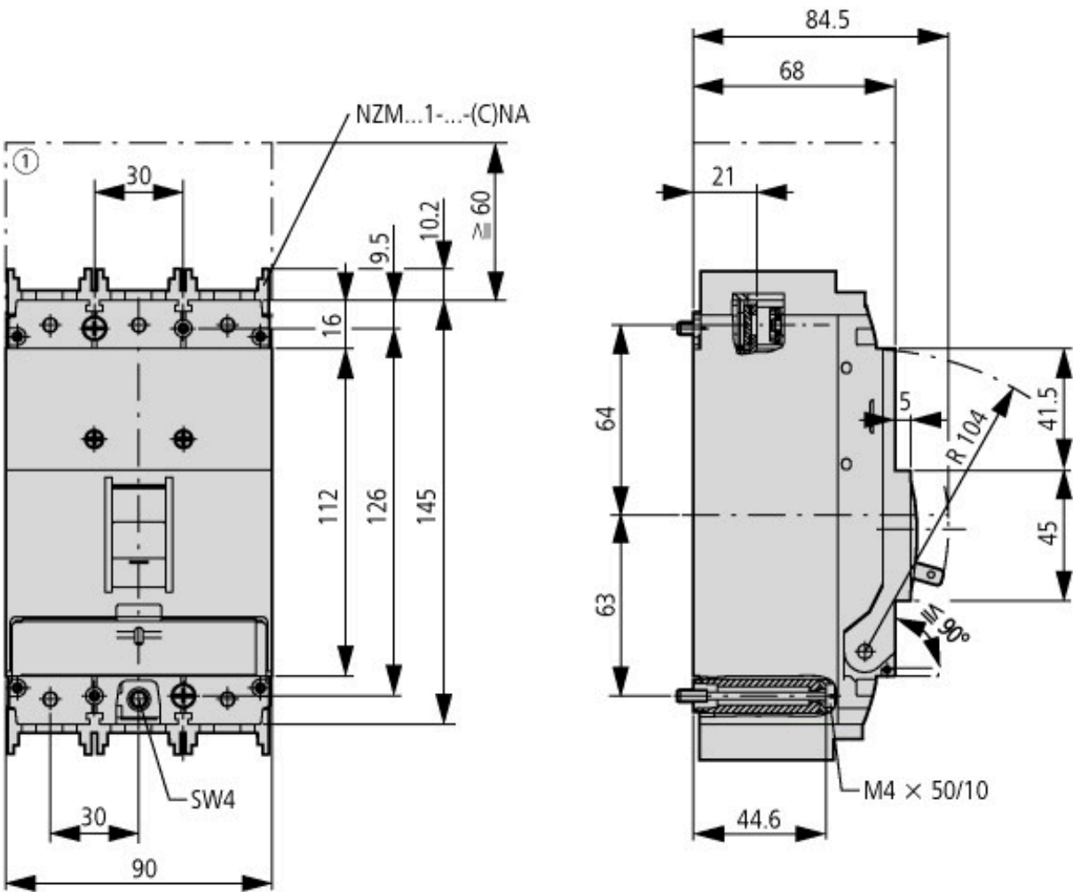
① Výfukový prostor, minimální vzdálenost od ostatních dílů
