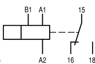
Označení přívodu podle EN 50042
