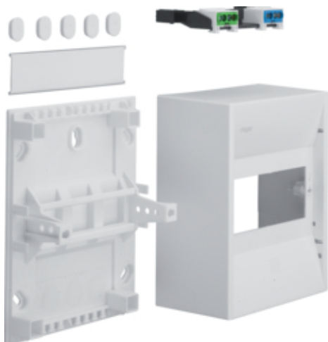
Minirozvodnice, IP30, 6 mod.
