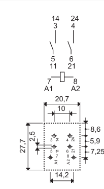
56.42-0300 pohled ze strany vývodů
