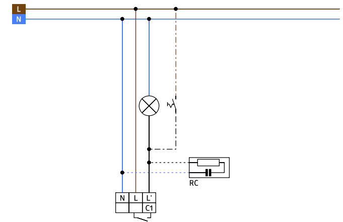
Schéma zapojení
