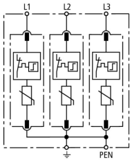
Schéma vnitřního zapojení DG M TNC 275
